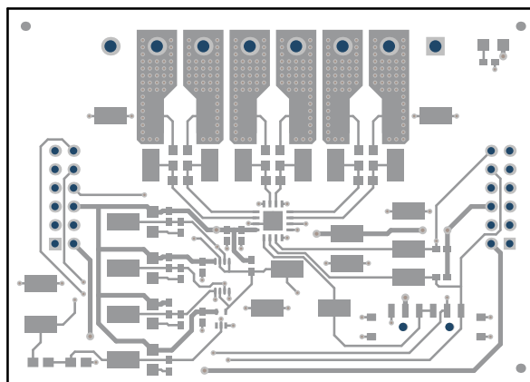
Figure 4-4. Top Layer
