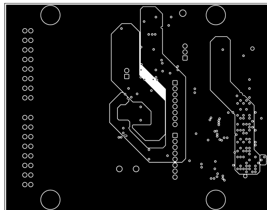
Figure 4-9. SIG Layer
