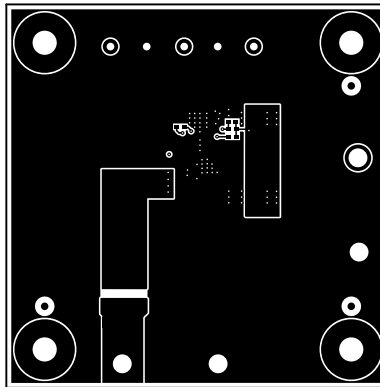
Figure 4-6. EVM Bottom Copper Layer
