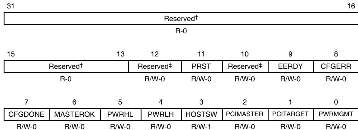
Figure B–235. PCI Interrupt Enable Register (PCIIEN)
