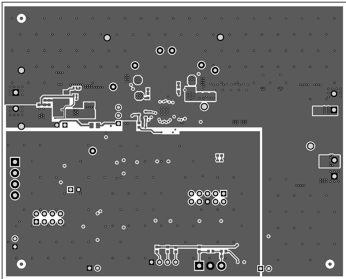
Figure 3-6. PCB Layer 4
