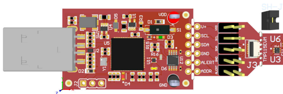
TMP115EVM
