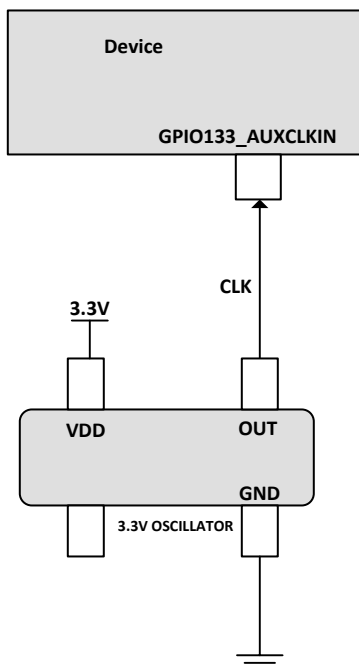
Figure 3-9. AUXCLKIN
