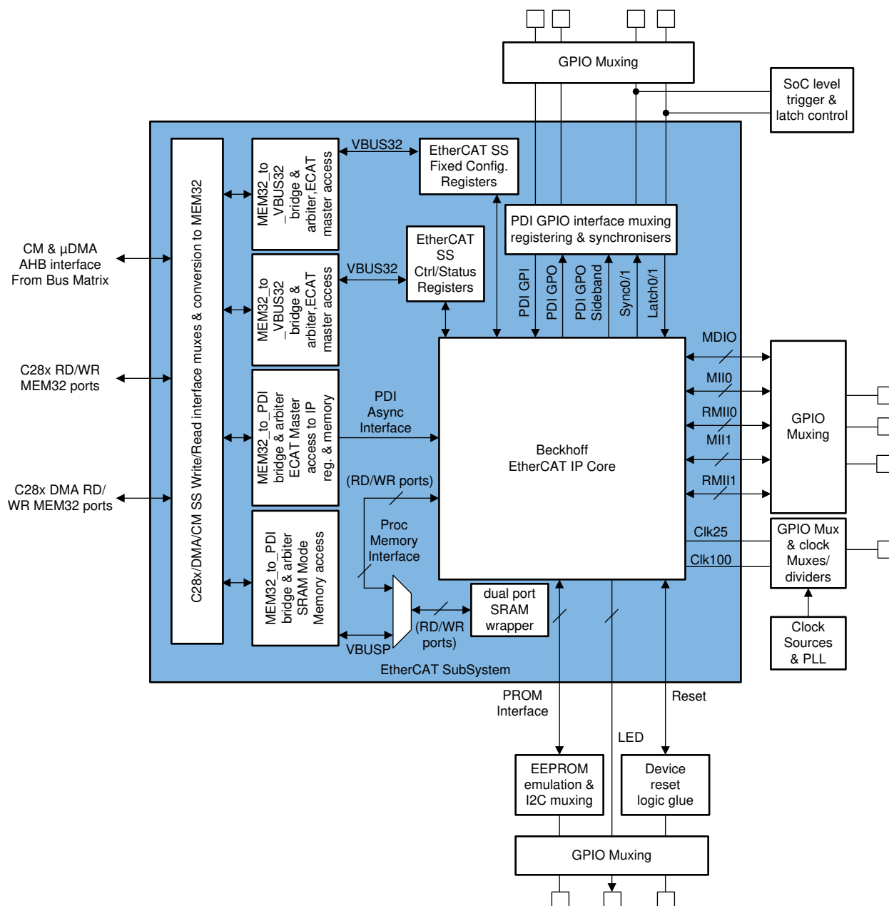
Figure 31-9. ESCSS Wrapper
