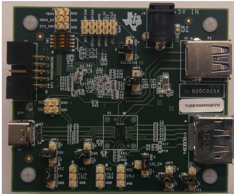
Figure 1. TUSB1064RNQ EVM
