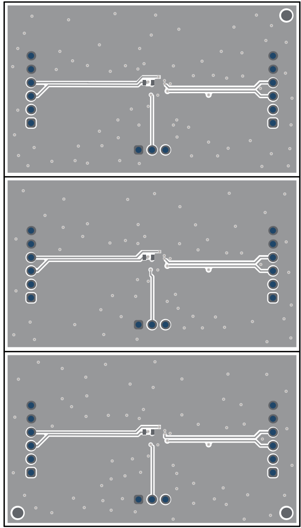
Figure 4-6. Bottom Layer
