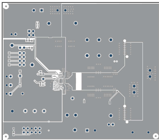
Figure 5-4. TPS544B27EVM Top Layer
