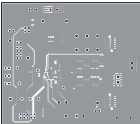
Figure 5-6. TPS544B27EVM Layer 3
