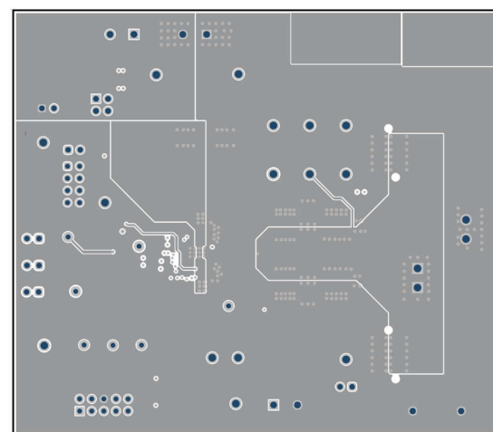
Figure 5-7. TPS544B27EVM Layer 4
