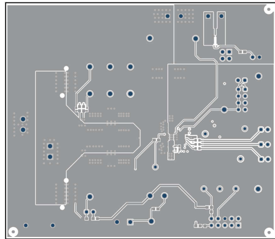
Figure 5-9. TPS544B27EVM Bottom Layer
