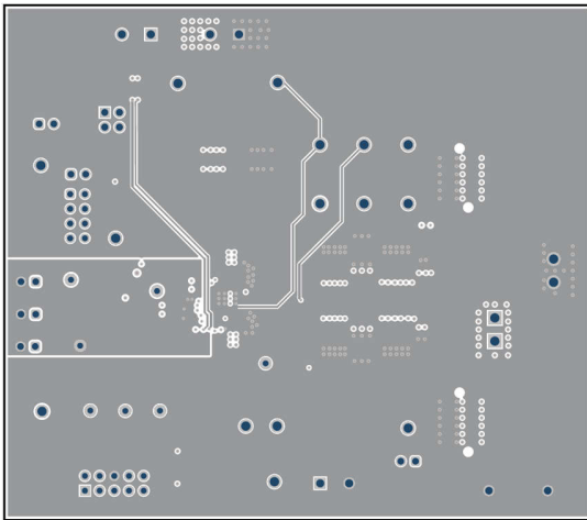
Figure 5-8. TPS544B27EVM Layer 5
