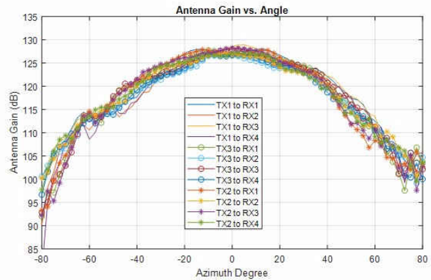
62 – 64 GHz
