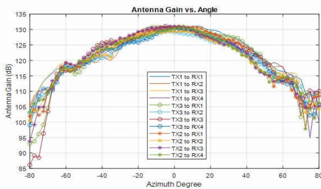
60 – 62 GHz
