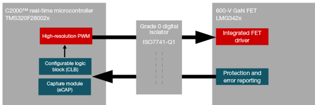
그림 4. C2000 MCU와 TI GaN 장치를 인터페이스하는 데 필요한 유일한 부품.
