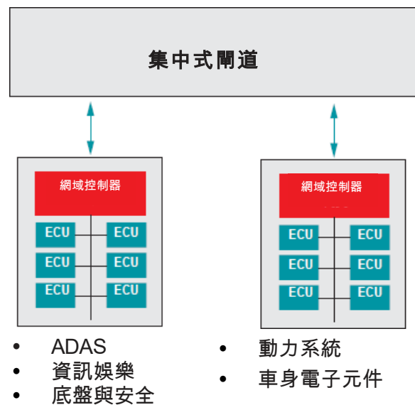
圖 1。SoC 架構範例，具備集中式閘道與兩個網域閘道。
