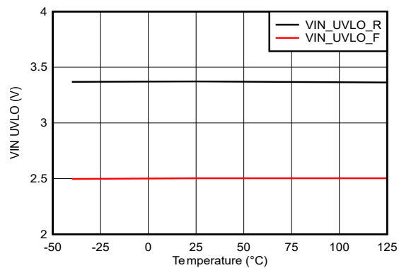
Figure 5-7. VIN UVLO
