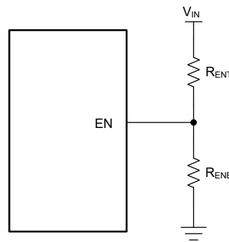
Figure 6-2. V_{IN} UVLO Using the EN Pin
