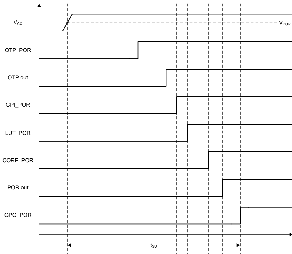
Figure 7-22. POR Sequence
