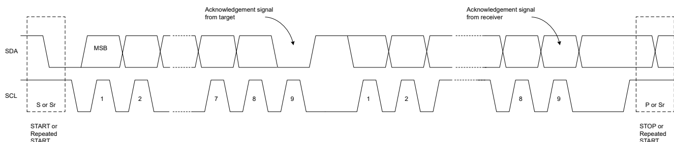
Figure 6-8. Byte Format
