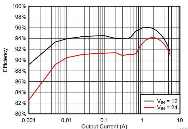
LMS3655-Q1 Efficiency: V_{\text{OUT}} = 5\text{ V}
