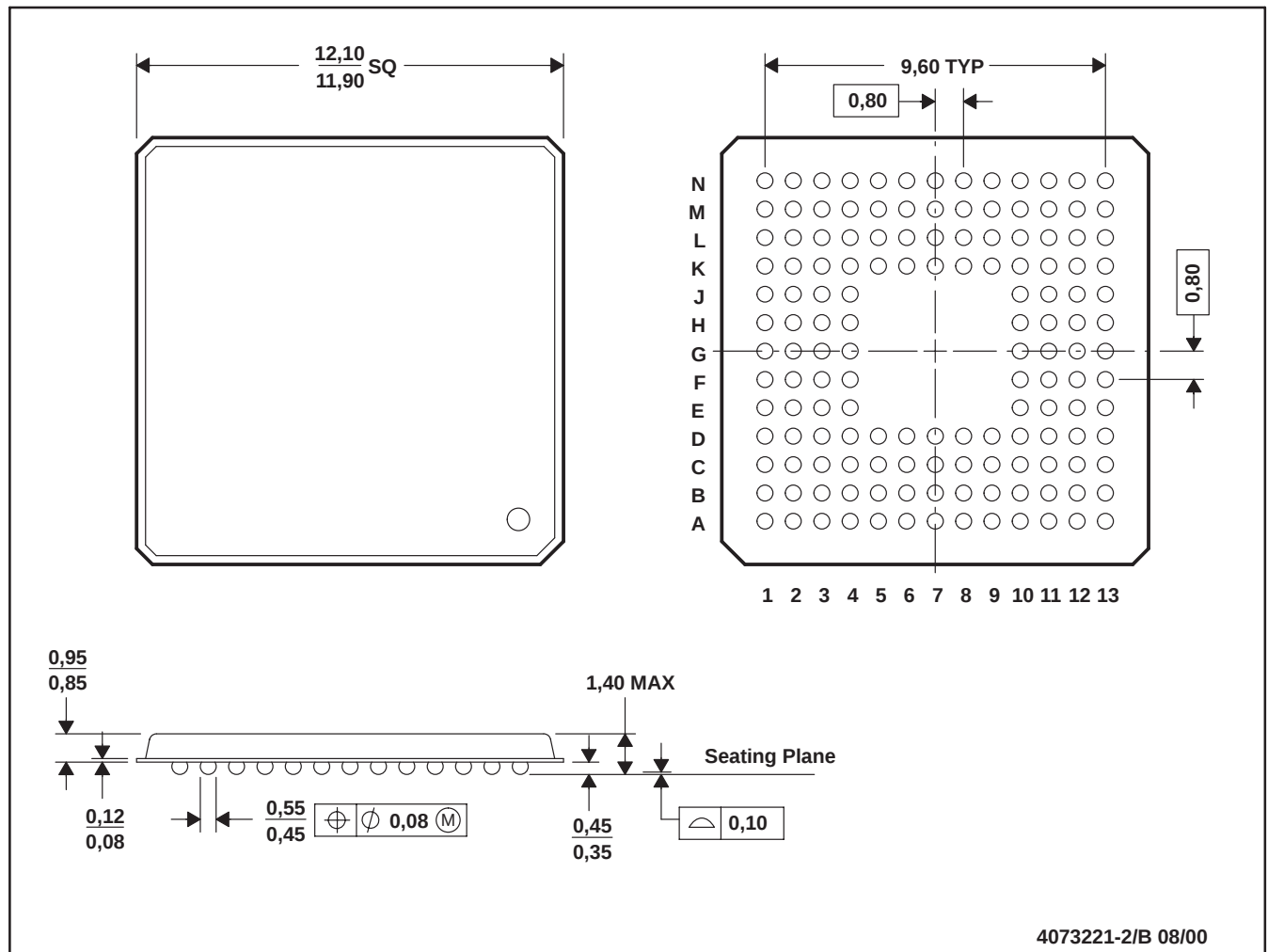
GGU (S-PBGA-N144)
