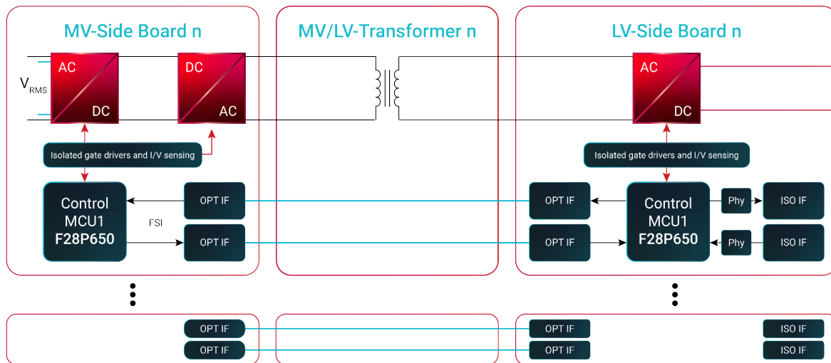
图 4. 採用 AC/DC 與隔離式 DC/DC 的轉換單元架構
