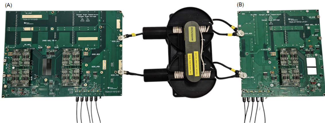
圖 5. 5050kW SiC 式模組化 SST，在中電壓 (A) 與低電壓 (B) PCB 間採用塑膠光纖介面
