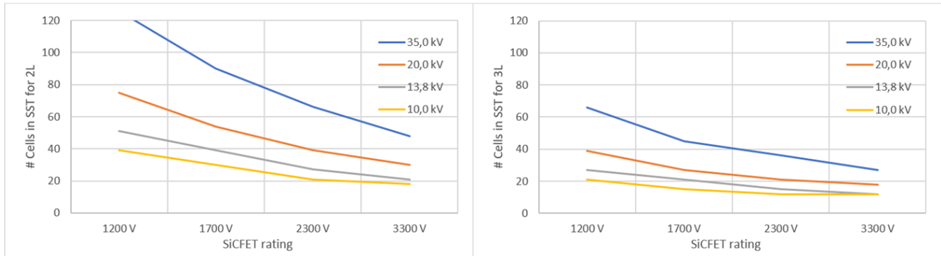
圖 3. 基於 SiC 額定值的 2L 和 3L 轉換單元的單元擴展
