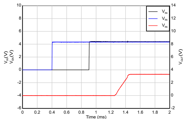
図 5-37. シーケンスによる起動 (EN 後の V_{IN} )
