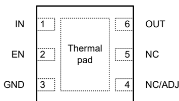
図 4-1. DRV パッケージ (固定/可変)、6 ピン WSON (上面図)
