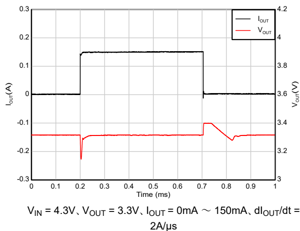
図 5-42. 負荷過渡応答 (0mA~150mA)
