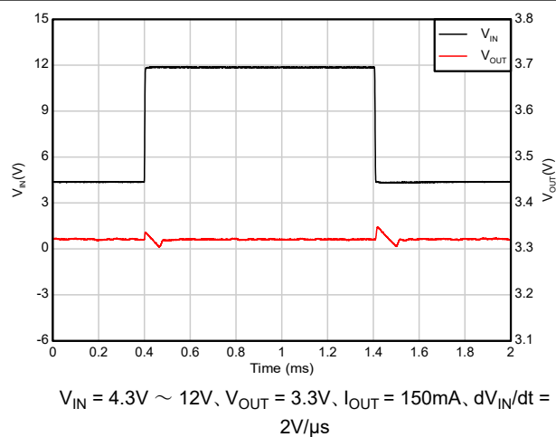
図 5-39. ライン過渡応答 (4.3V ~ 12V)
