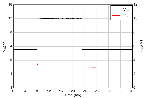
図 5-48. コールドクランク回復
