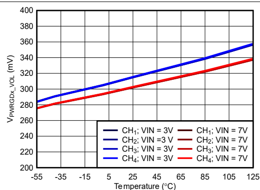
図 6-82. パワー グッド出力 Low 電圧と温度との関係
