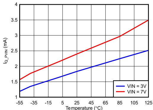
図 6-57. PVIN シャットダウン電流と温度との関係
