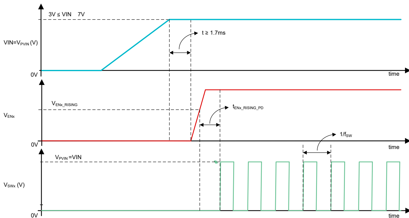
図 7-3. ENx が PVIN = VIN から独立して駆動されたときの立ち上がりリネーブル伝搬遅延 ( t_{ENx\_RISING\_PD} )
