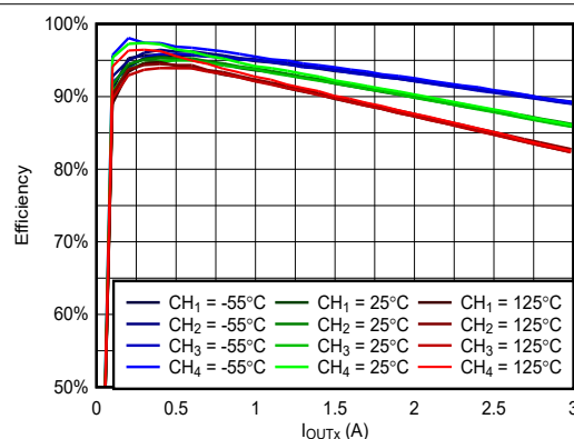
図 6-4. 効率と負荷との関係 (VIN = 3.3V、VOUTX = 1.8V、fSW = 100kHz)
