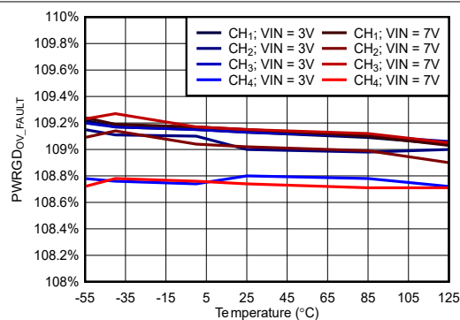
図 6-80. PWRGD フォルトの VSNSx 立ち上がりスレッシュホールドと温度との関係
