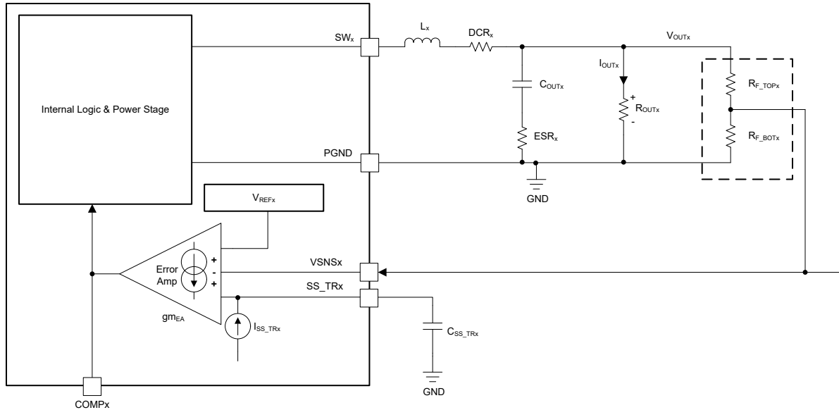
図 8-1. 抵抗分圧器による V_{OUTx} のプログラミング
