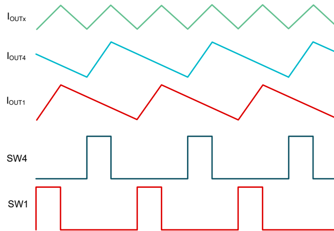
図 9-17. SW1 と SW4 の並列におけるインダクタ リップル電流
