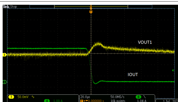
図 9-4. V_{OUT1} での全負荷立ち下がりステップ
