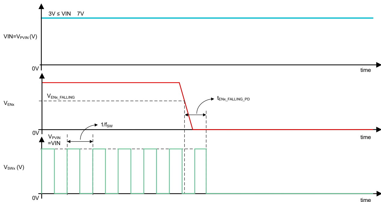
図 7-4. 立ち下がリリネーブル伝搬遅延 ( t_{ENx\_FALLING\_PD} )
