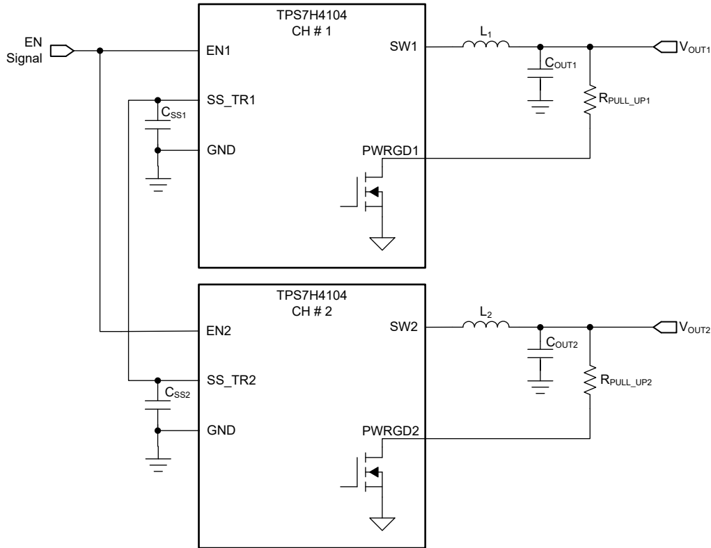
図 8-12. レシオメトリック起動シーケンス
