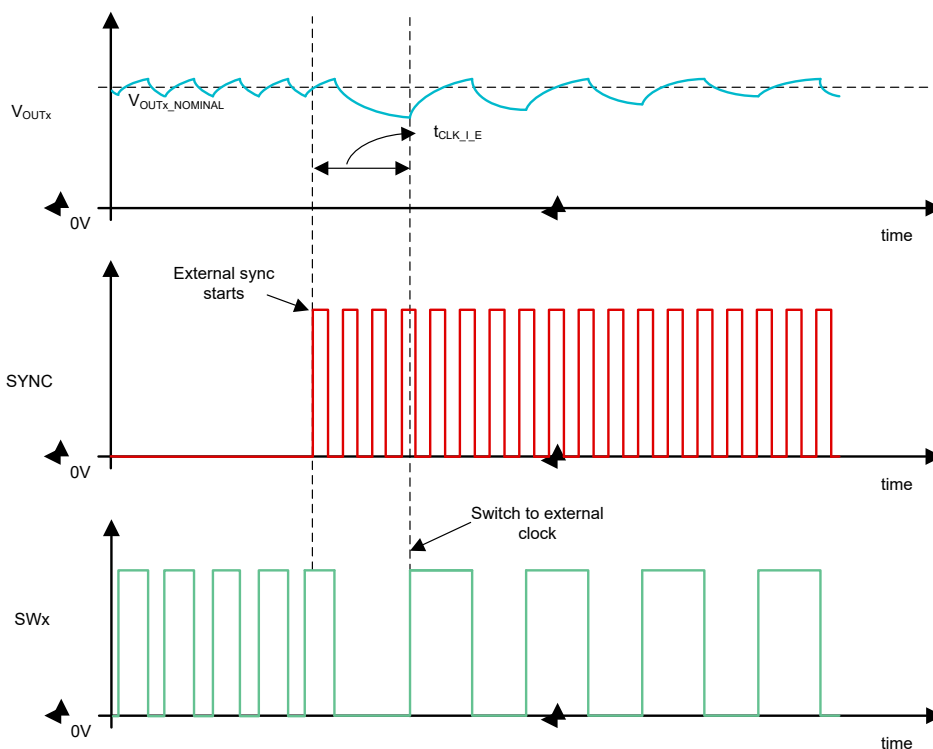
図 8-9. 内部クロックから外部クロックへの遷移
