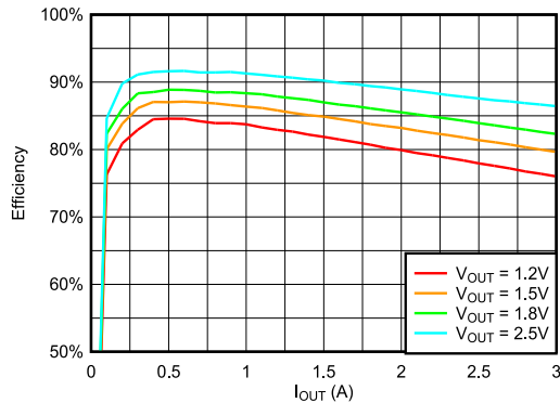
図 6-43. VIN = 3.3V、f SW = 1MHz、チャネル #1、25°C における V OUT 全域での効率対負荷
