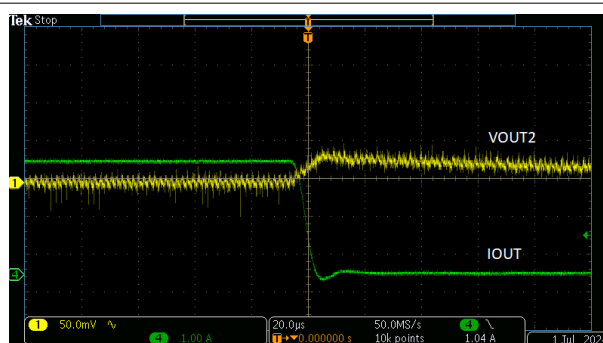
図 9-6. V_{OUT2} での全負荷立ち下がりステップ
