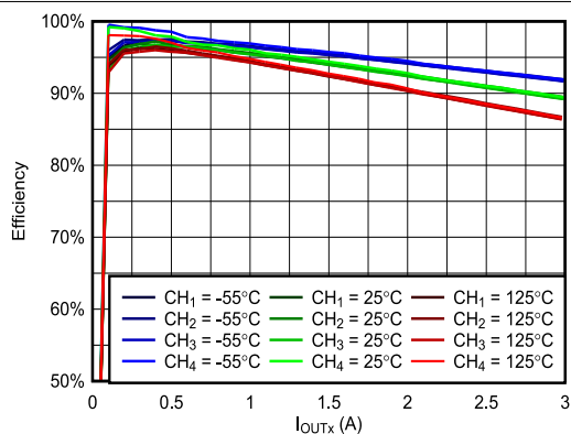
図 6-5. 効率と負荷との関係 (VIN = 3.3V、VOUTX = 2.5V、fSW = 100kHz)
