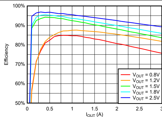
図 6-6. VIN = 3.3V、fSW = 100kHz、チャネル #1、25°C における VOUT 全域での効率対負荷
