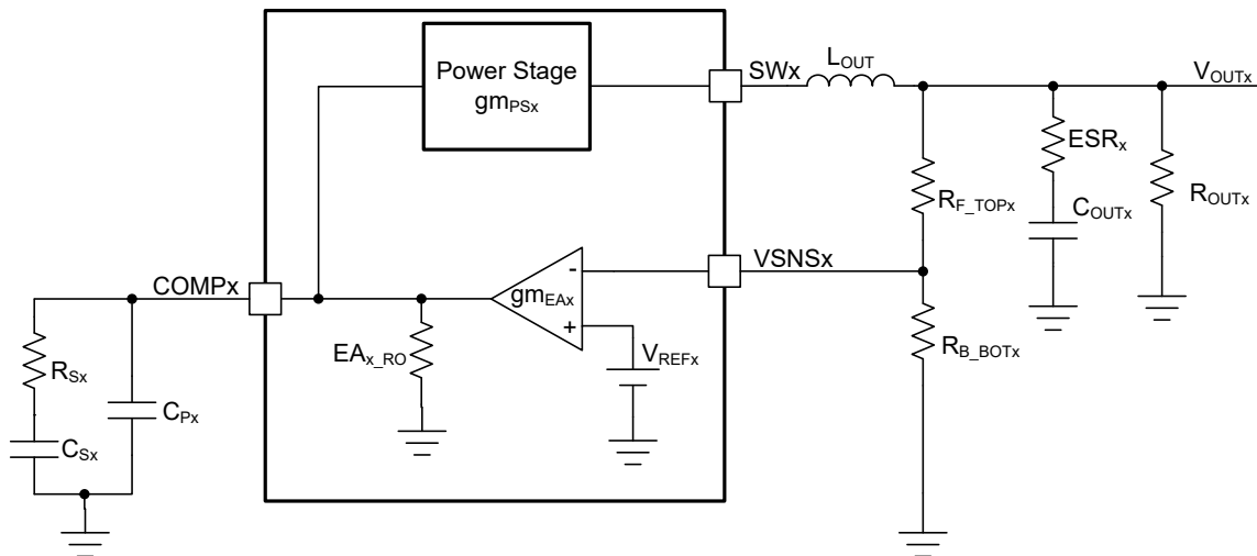
図 8-17. ループ応答の小信号モデル
