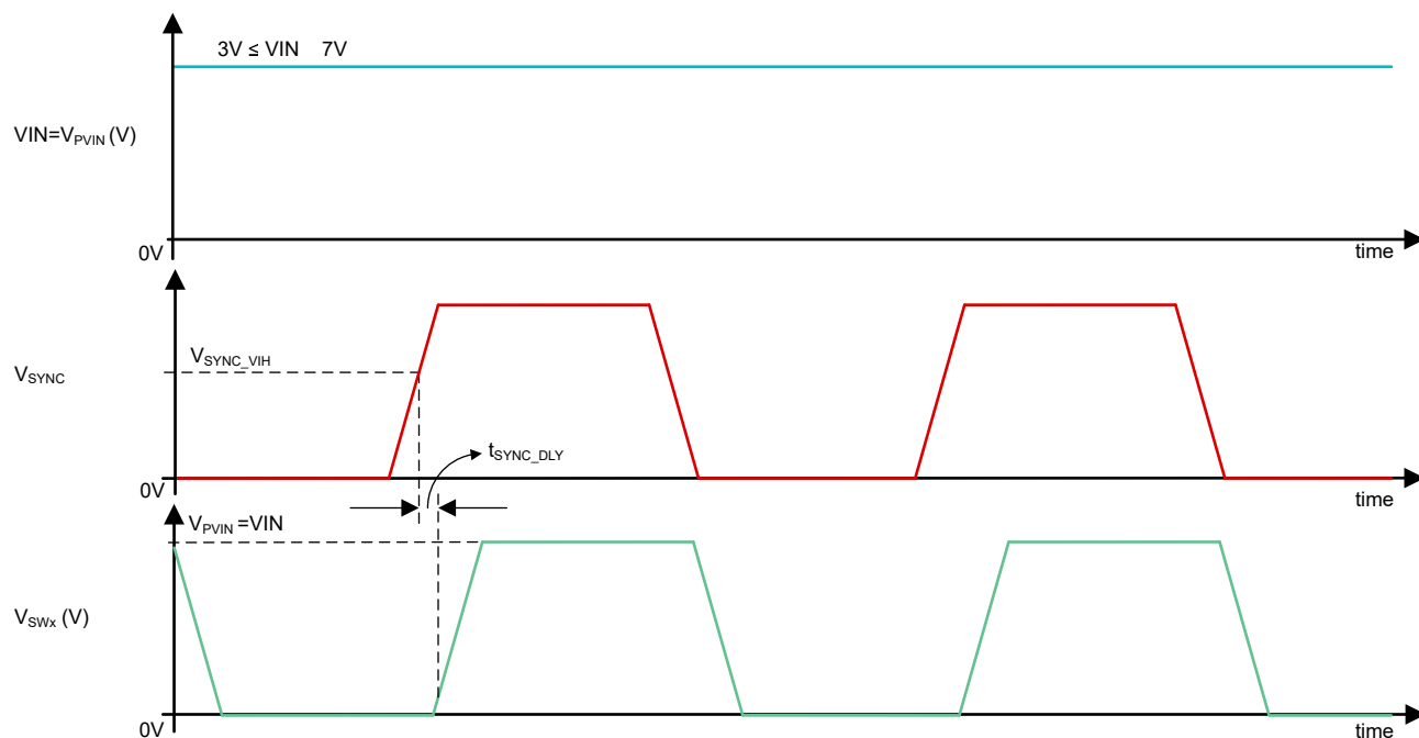
図 7-5. SYNC からスイッチまでの遅延 ( t_{\text{SYNC\_DLY}} )
