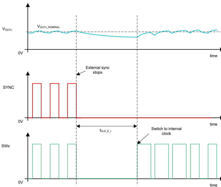
図 8-10. 外部から内部へのクロック遷移
