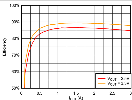
図 6-51. VIN = 7V、f SW = 1MHz、チャネル #1、25°C における V OUT 全域での効率対負荷
