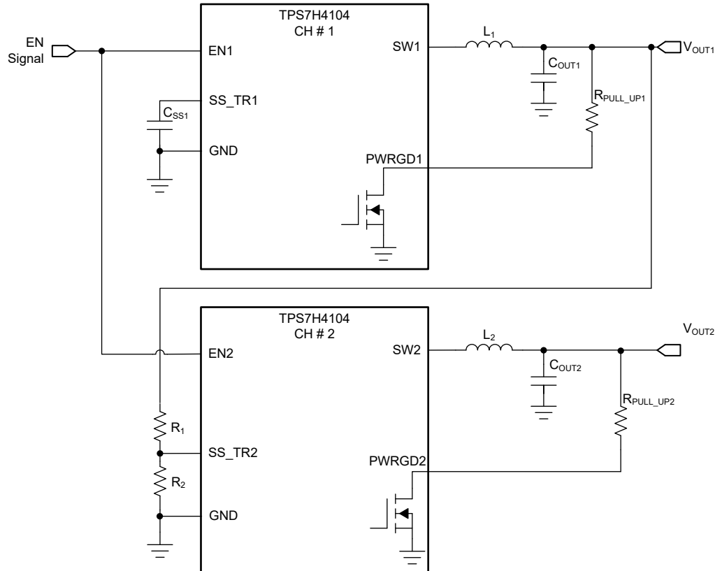
図 8-13. レシオメトリックおよび同時起動シーケンス
