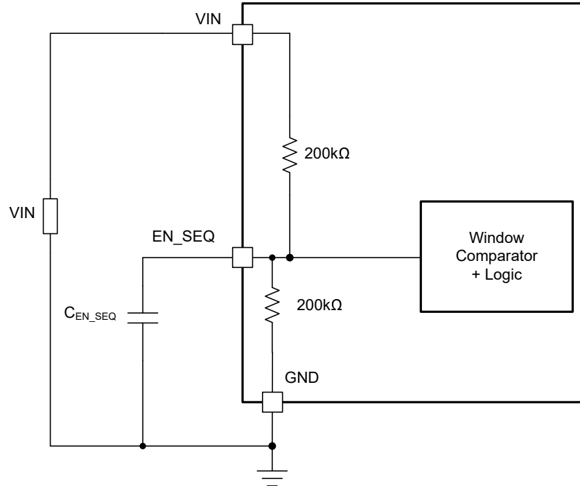
図 8-4. EN_SEQ の内部公称インピーダンス
