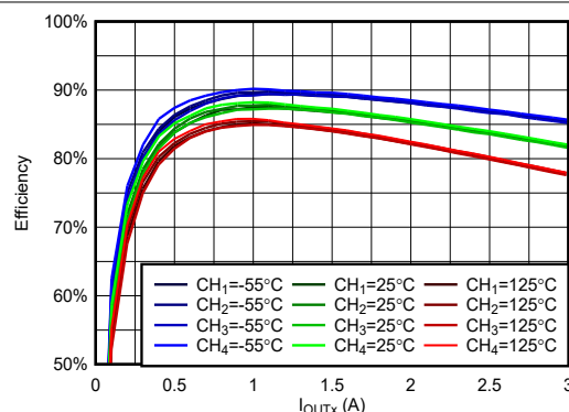
図 6-2. 効率と負荷との関係 (VIN = 3.3V、VOUTX = 1.2V、fSW = 100kHz)
