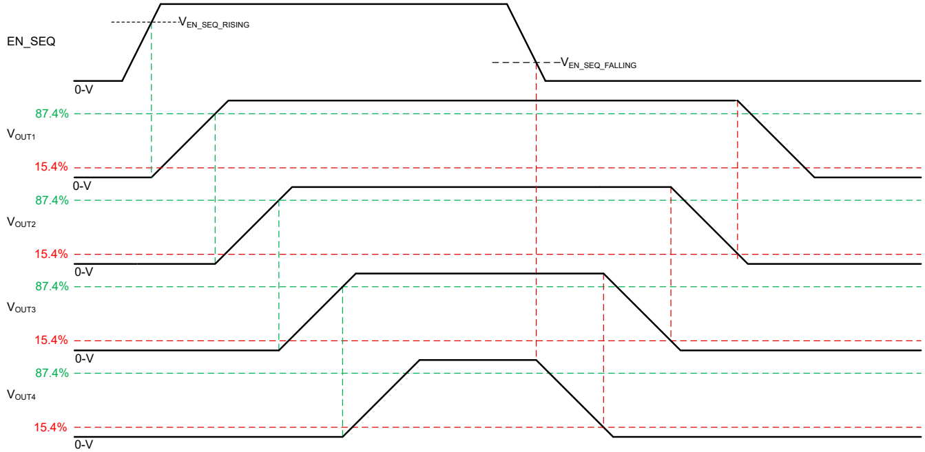
図 8-3. シーケンスのアップ/ダウン
