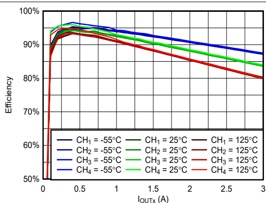
図 6-3. 効率と負荷との関係 (VIN = 3.3V、VOUTX = 1.5V、fSW = 100kHz)
