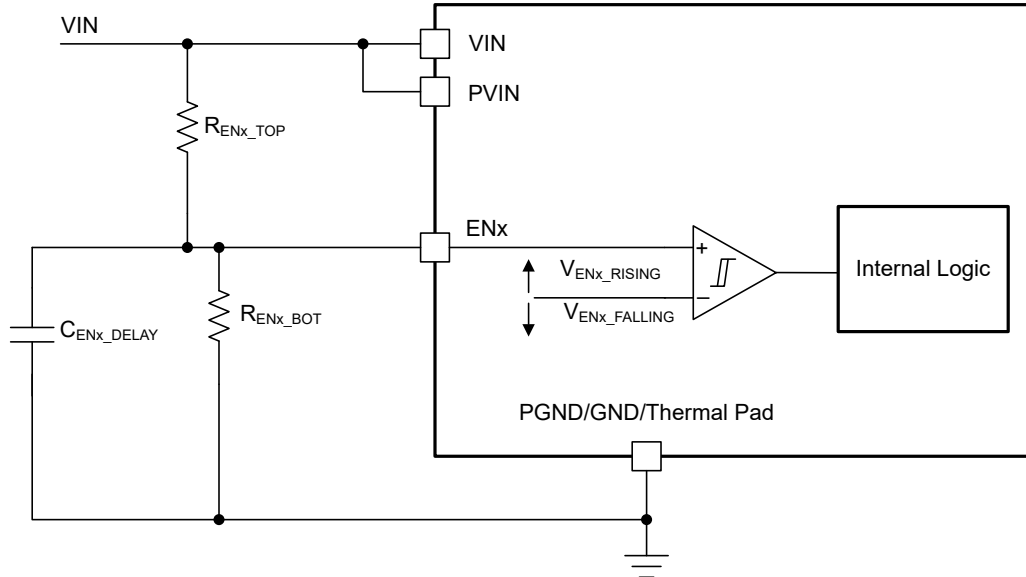
図 8-2. ENx と抵抗分圧器を使用した外部 UVLO
