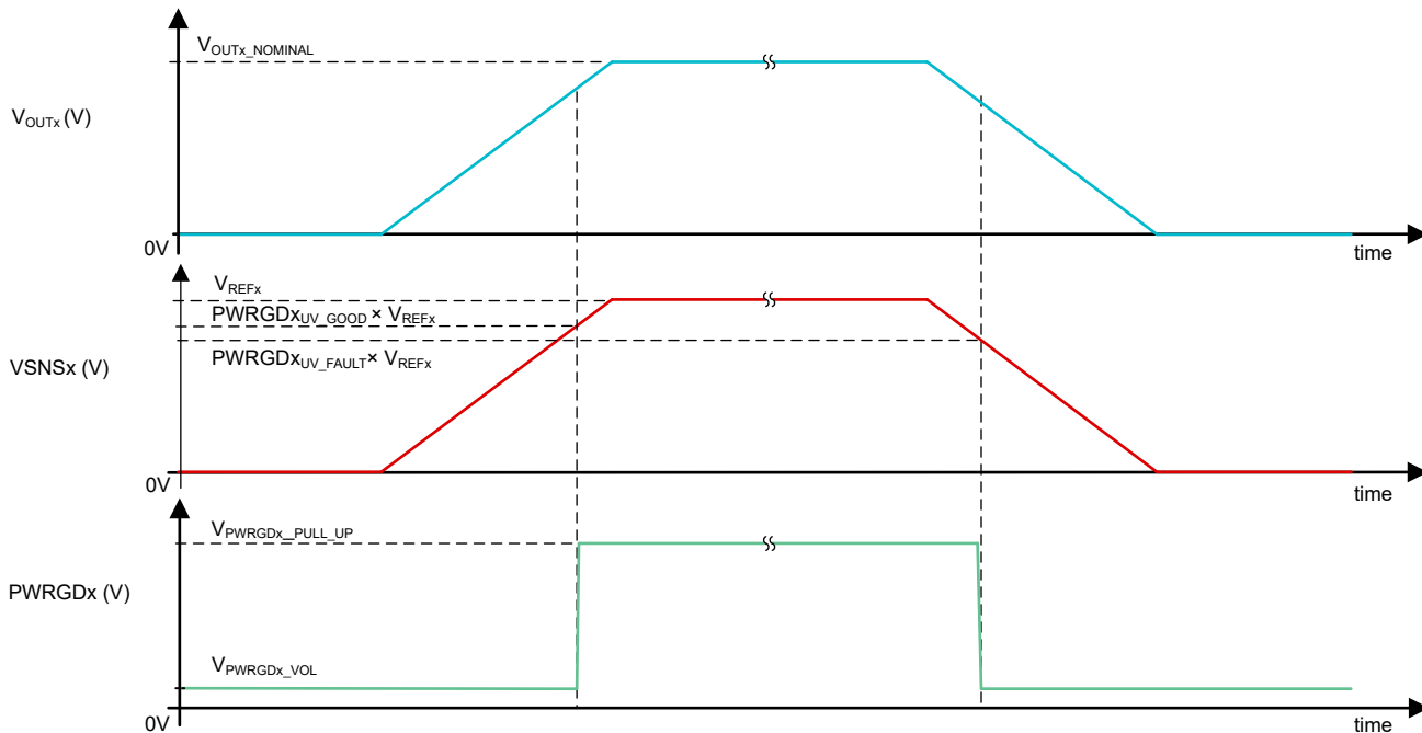
図 8-5. PWRGDx 低電圧 (UV) スレッショルド
