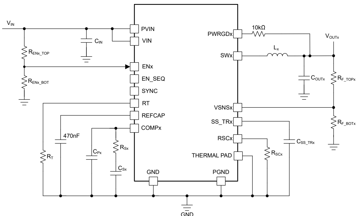
図 9-1. 代表的なアプリケーション回路図
