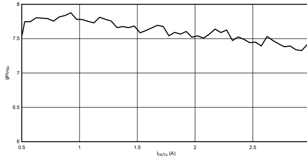
図 8-18. gm_{PSx} と I_{OUTx} の関係 ( P_{VIN} = V_{IN} = 5V , T_A = 25^\circ C )
