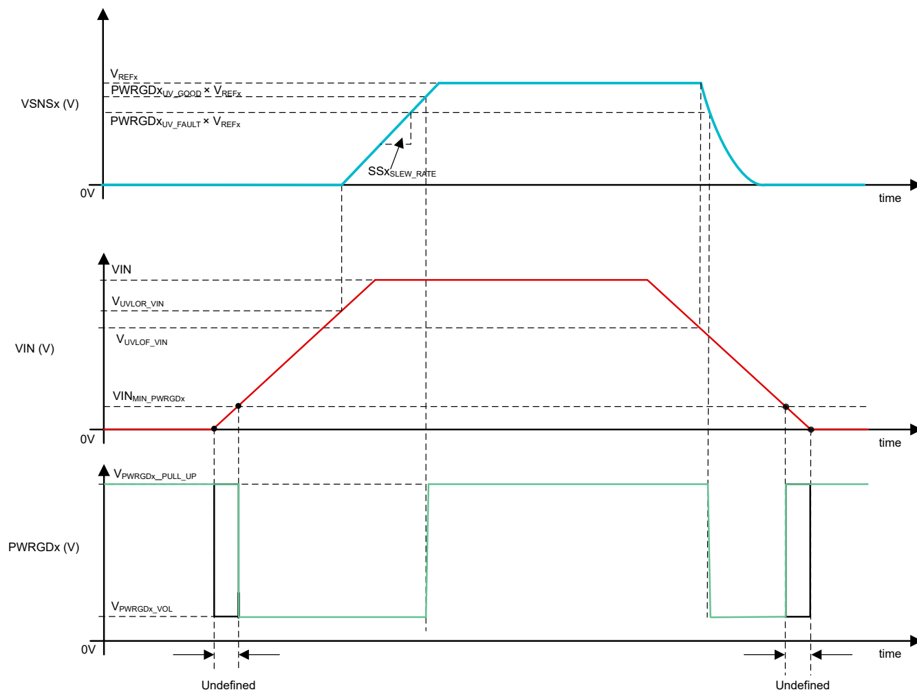
図 8-7. V_{IN} > V_{IN\_MIN\_PWRGDx} の後で有効な状態になる PWRGDx
