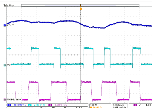
図 9-25. 外部クロック TPSM8287B30HAPx への同期
