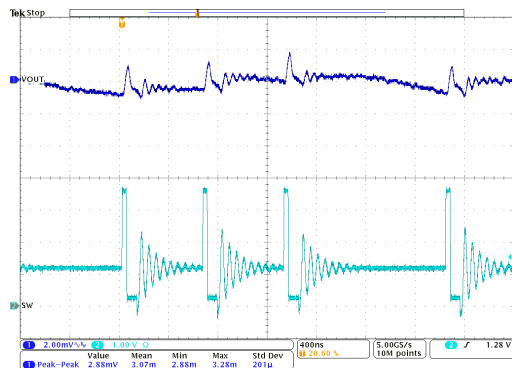
図 9-24. PFM-DCM 動作 TPSM8287B30HAPx
