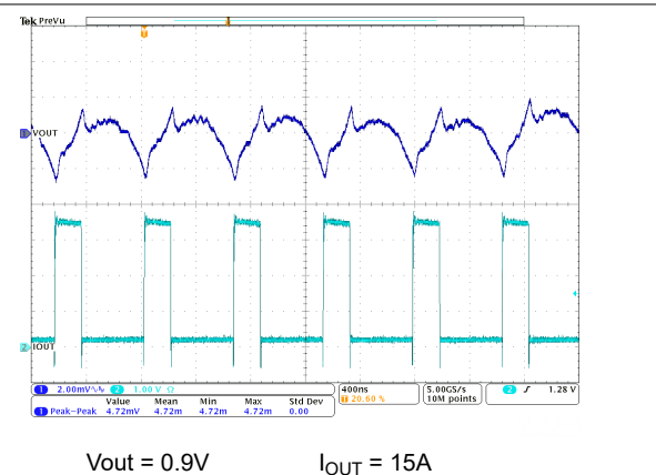
図 9-22. PWM-CCM 動作 TPSM8287B30HAPx
