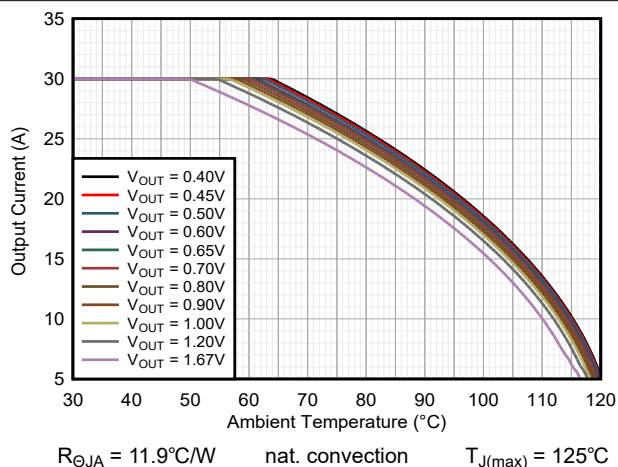
図 9-33. 安全動作領域 TPSM8287B30xx V_{IN} = 5.0V
