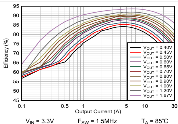
図 9-11. 効率 TPSM8287B30xx PSM
