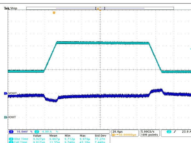
図 9-44. 負荷過渡 TPSM8287B30HAPx
