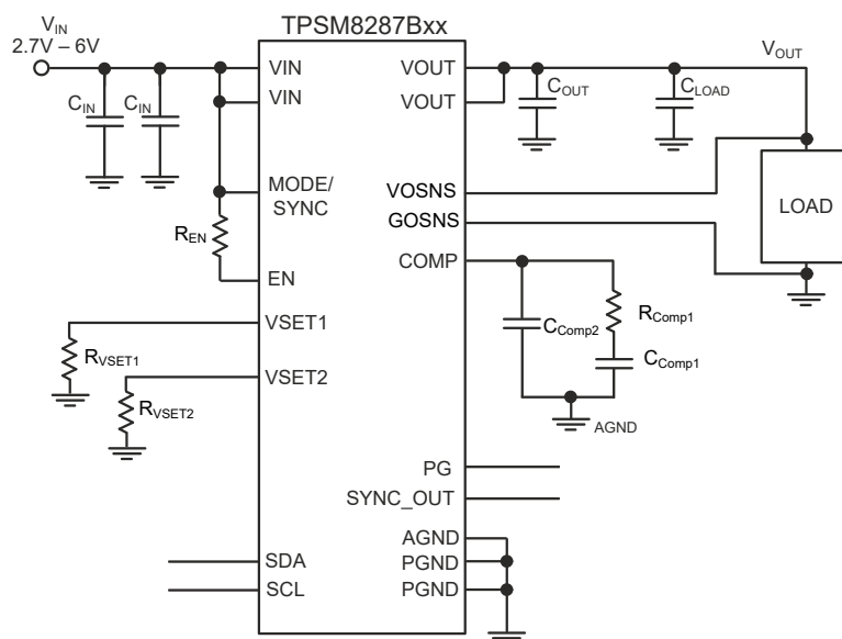
TPSM8287Bxx の概略回路図
