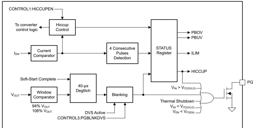
図 7-16. パワーグッド機能のブロック図 (スタンドアロン、プライマリ デバイス)
