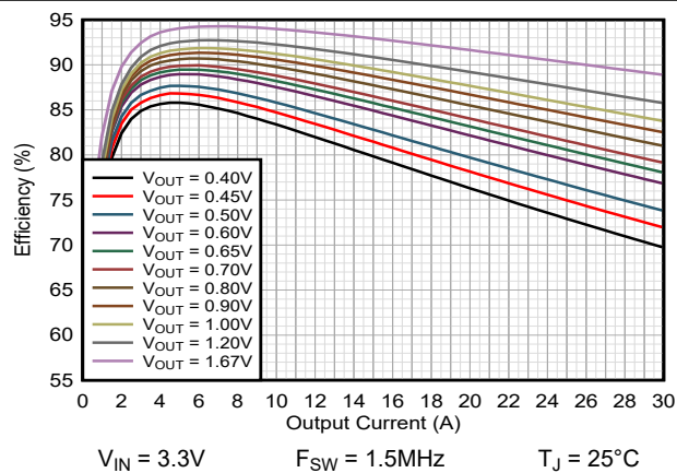
図 9-4. 効率 TPSM8287B30xx FPWM
