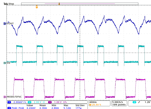
図 9-25. 外部クロック TPSM8287B30HAPx への同期
