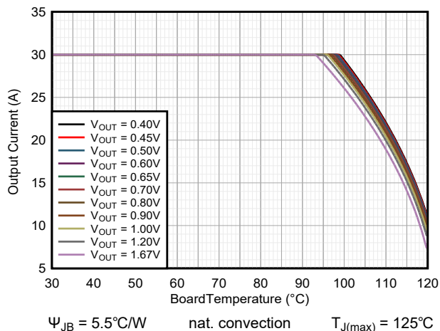
図 9-35. 安全動作領域 TPSM8287B30xx V_{IN} = 5.0V
