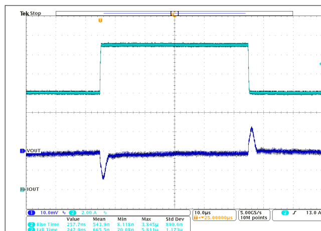
図 9-43. 負荷過渡 TPSM8287B30HAPx
