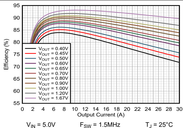
図 9-6. 効率 TPSM8287B30xx FPWM
