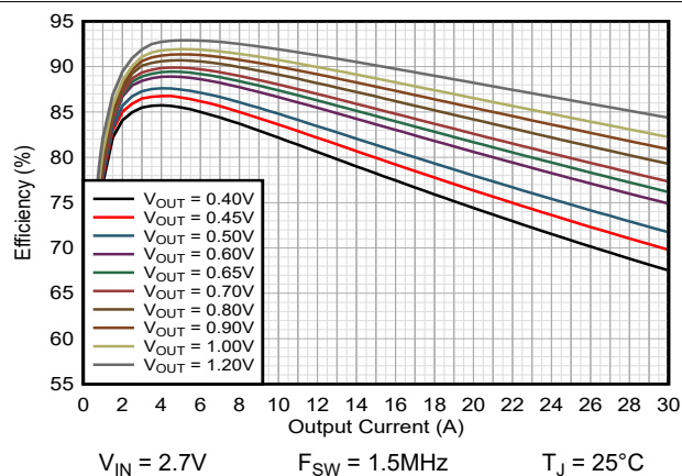
図 9-2. 効率 TPSM8287B30xx FPWM
