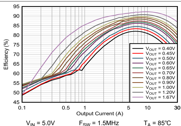
図 9-13. 効率 TPSM8287B30xx PSM
