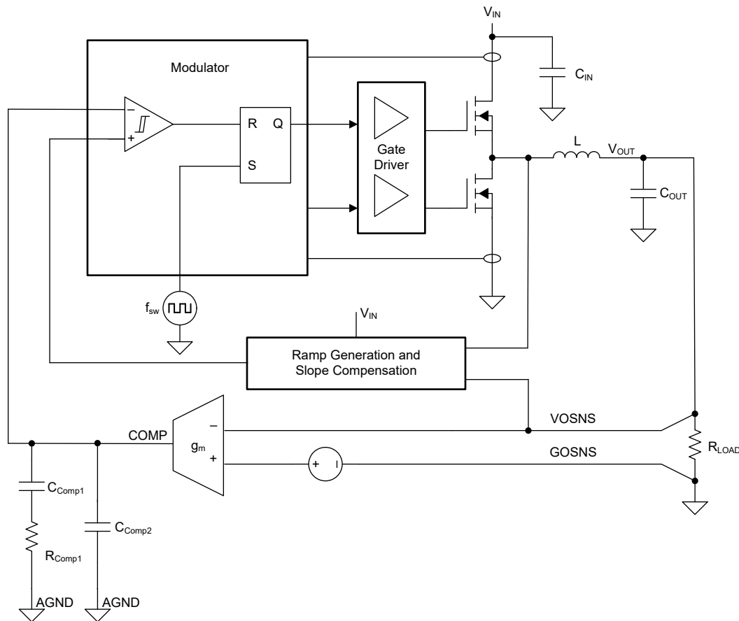
図 7-1. 固定周波数の DCS-Control トポロジ (簡略図)
