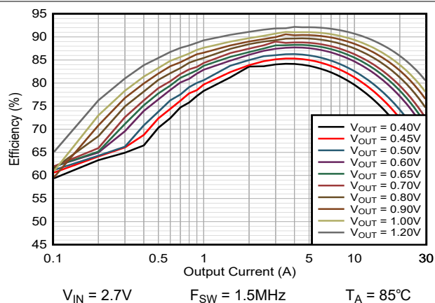
図 9-9. 効率 TPSM8287B30xx PSM
