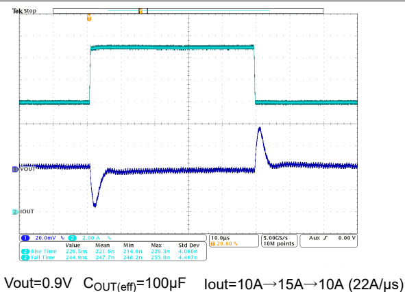
図 9-20. 負荷過渡 TPSM8287B30HAPx
