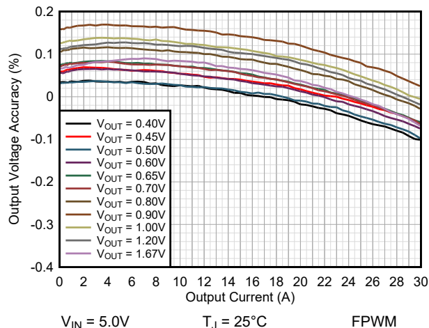
図 9-18. 負荷レギュレーション TPSM8287B30xx
