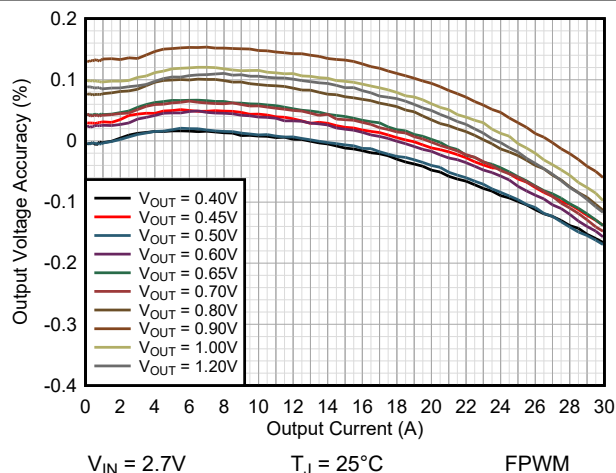
図 9-14. 負荷レギュレーション TPSM8287B30xx
