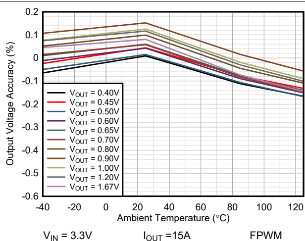
図 9-17. Vout の精度と温度との関係 TPSM8287B30xx
