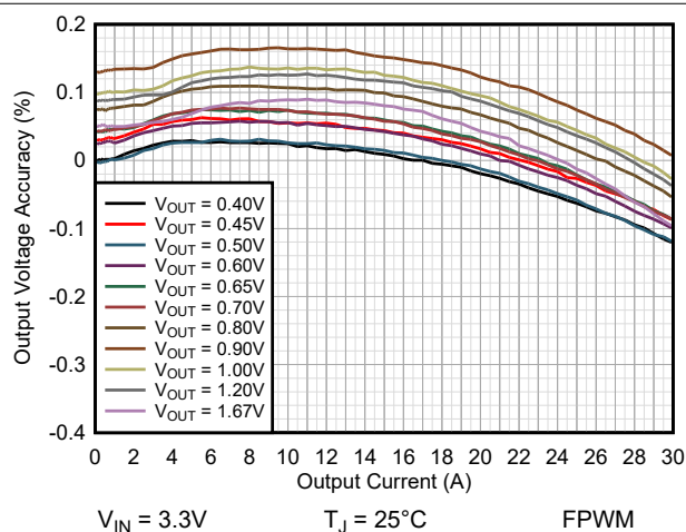
図 9-16. 負荷レギュレーション TPSM8287B30xx
