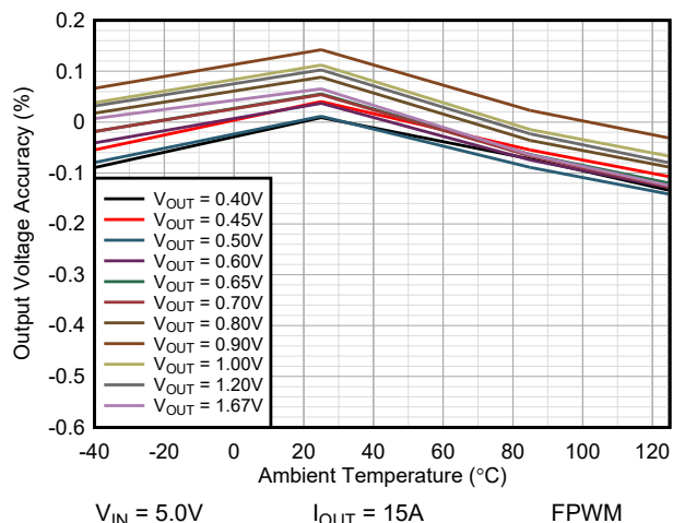
図 9-19. Vout の精度と温度との関係 TPSM8287B30xx
