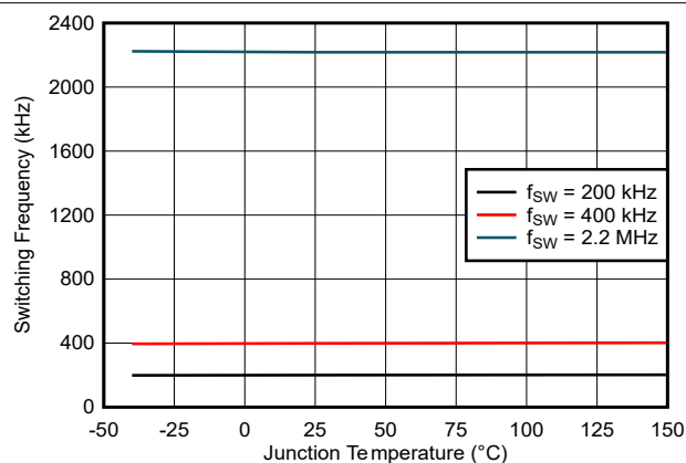
図 6-5. SYNC により設定されるスイッチング周波数
