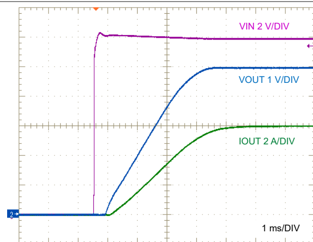
図 8-5. LM644x0-Q1 の起動、6A の抵抗性負荷
