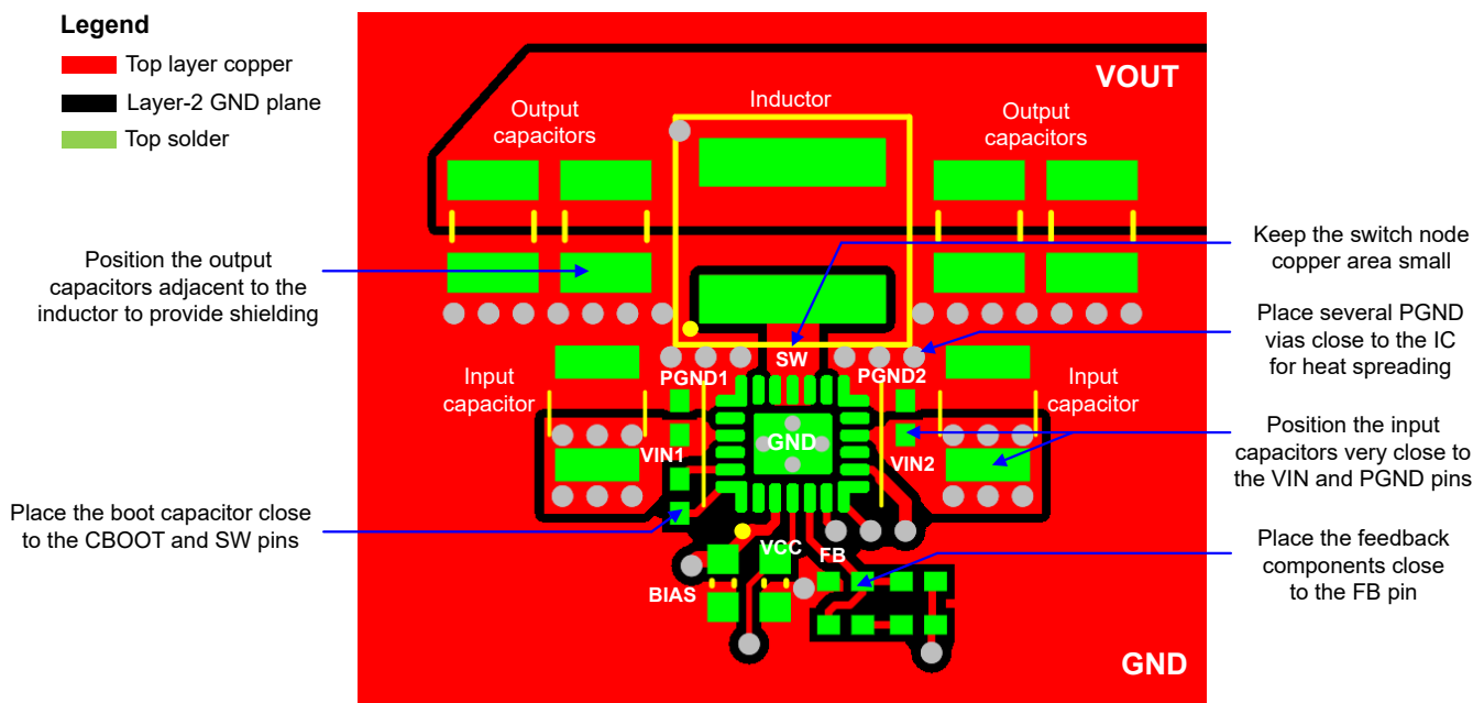
図 8-22. PCB のレイアウト例
