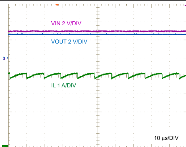
図 8-12. ドロップアウト時の LM644x0-Q1 の周波数フ ォールドバック、 V_{IN} = 3V
