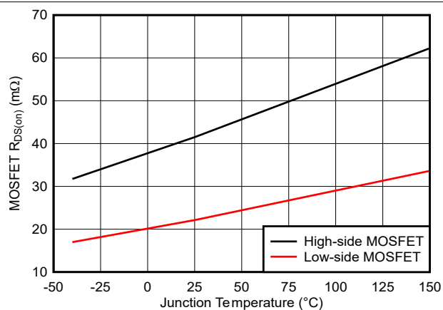
図 6-6. 下限側および上限側 MOSFET R_{DS(on)}
