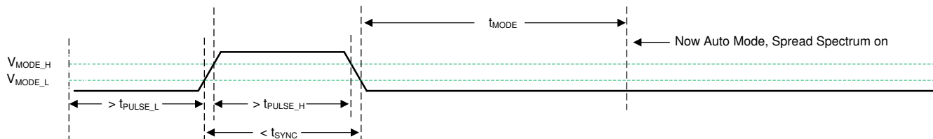
図 7-10. 同期モードから AUTO モードへの遷移
