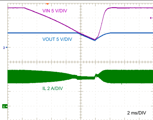
図 8-11. LM644x0-Q1 のライン過渡とドロップアウト からの回復
