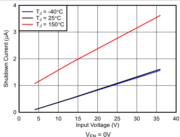
図 6-2. シャットダウン時の電源電流
