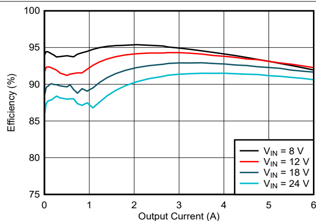
図 8-3. LM644x0-Q1 の効率
