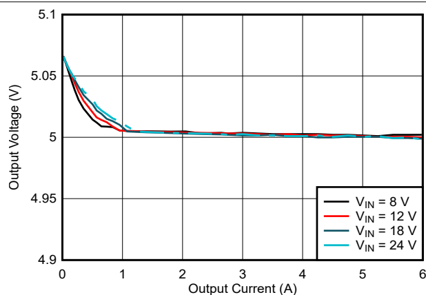
図 8-4. LM644x0-Q1 の負荷およびラインレギュレーション
