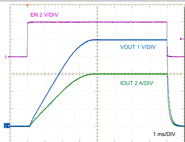
図 8-6. LM644x0-Q1 イネーブルのオン / オフ、6A の抵抗性負荷
