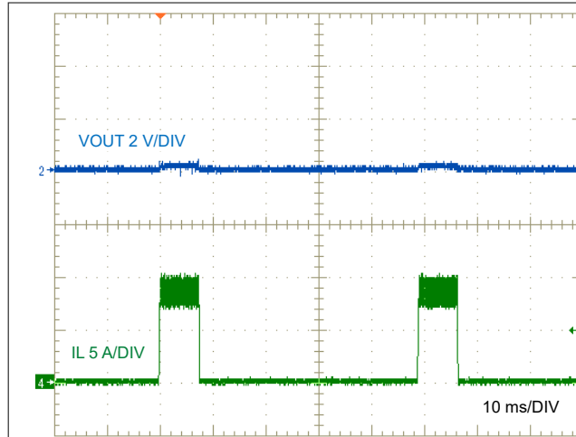
図 7-18. ヒカップ中のインダクタ電流バースト
