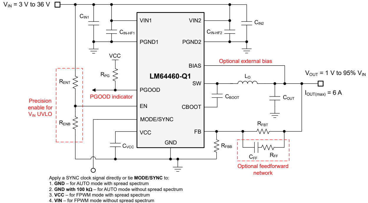
図 7-1. 入力電圧動作範囲が 3V ~ 36V の場合の LM64460-Q1 の回路図
