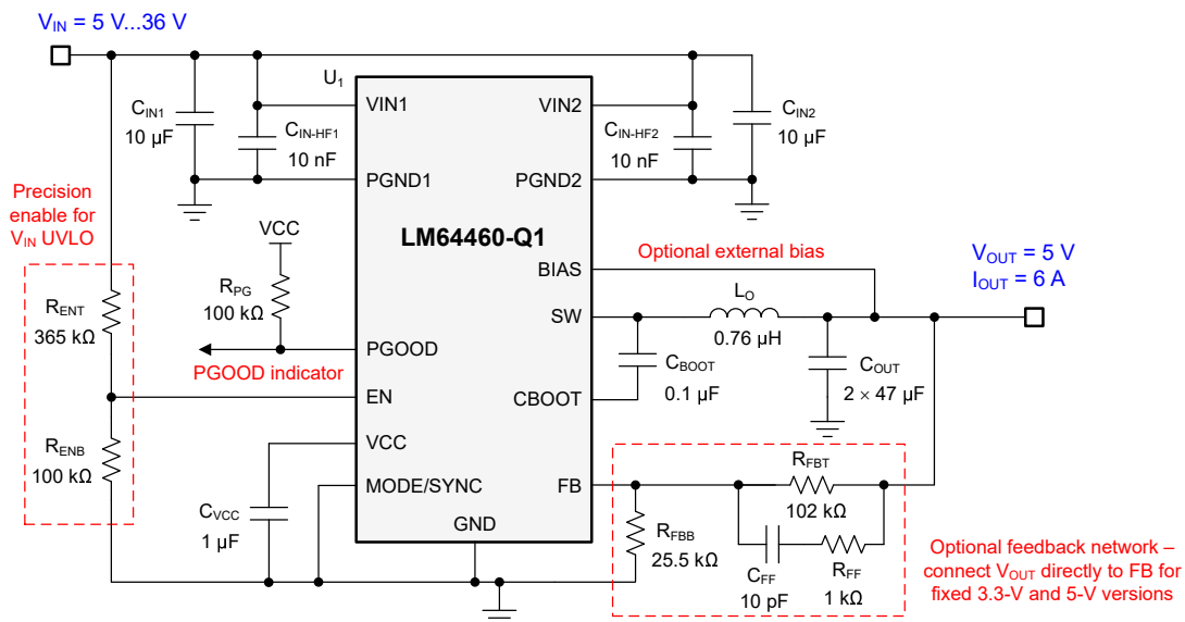
図 8-1. アプリケーション回路 1 - 5V、6A、2.1MHz
