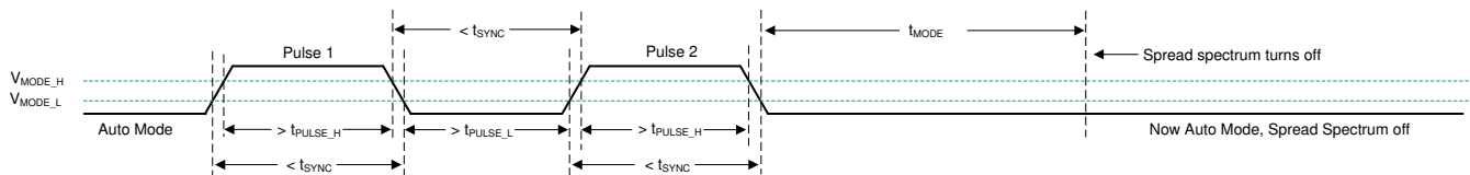
図 7-7. AUTO モードでのスペクトラム拡散の無効化
