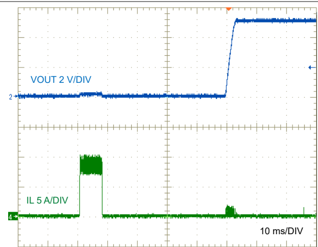
図 7-19. 短絡からの回復
