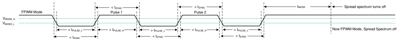
図 7-6. FPWM モードでのスペクトラム拡散の無効化
