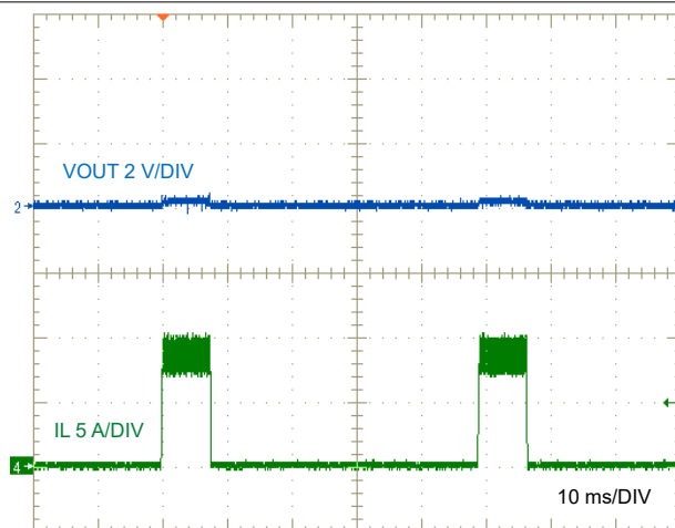
図 8-9. LM644x0-Q1 の短絡ヒカッ
