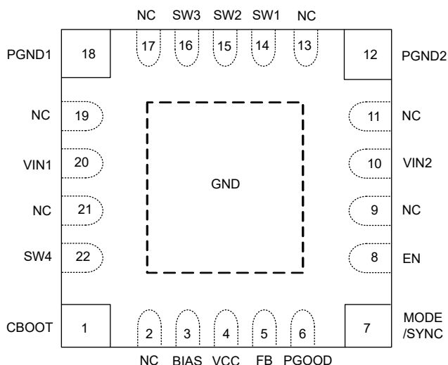
図 5-1. 22 ピン Enhanced HotRod™ VQFN-FCRLF RYF パッケージ (上面図)
