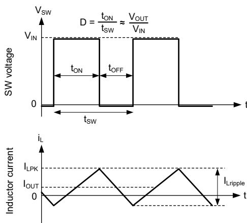
図 7-23. FPWM モード動作
