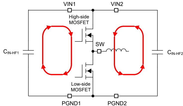
図 8-21. 入力電流ループ
