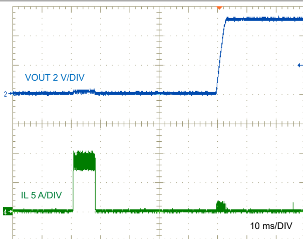
図 8-10. LM644x0-Q1 の短絡から無負荷への回復
