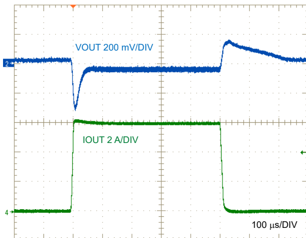
図 8-8. LM644x0-Q1 の負荷過渡、 I_{OUT} = 0A \sim 6A
