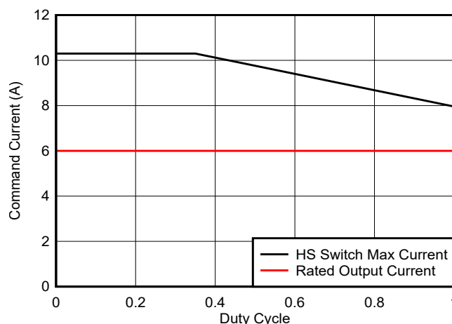
図 7-16. LM64460-Q1 の HS スイッチ最大電流はデューティ サイクルの関数
