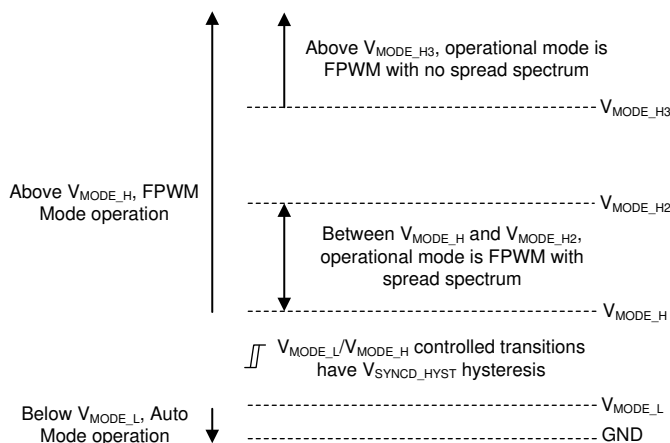
図 7-2. レベル依存モード選択設定
