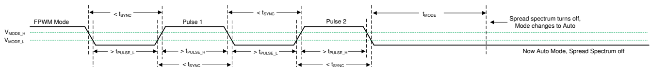
図 7-8. FPWM モードから自動モードへの遷移でのスペクトラム拡散の無効化
