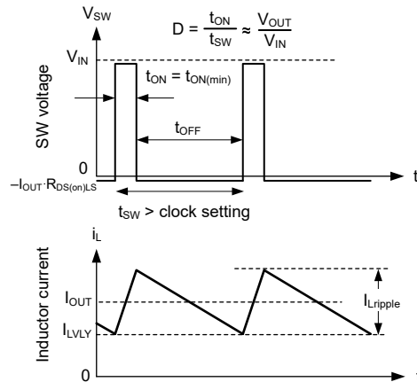
図 7-24. バレー電流動作
