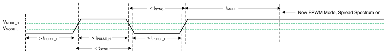
図 7-11. 同期モードから FPWM モードへの遷移
