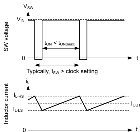
図 7-17. 電流制限波形
