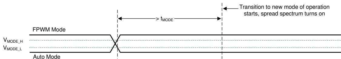
図 7-5. 自動モードと FPWM モードとの間の遷移
